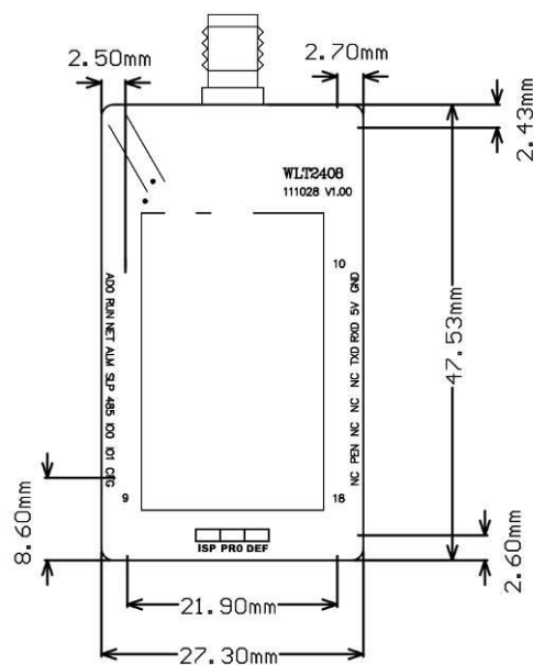
图 1-2 WLT2408Z 结构尺寸
