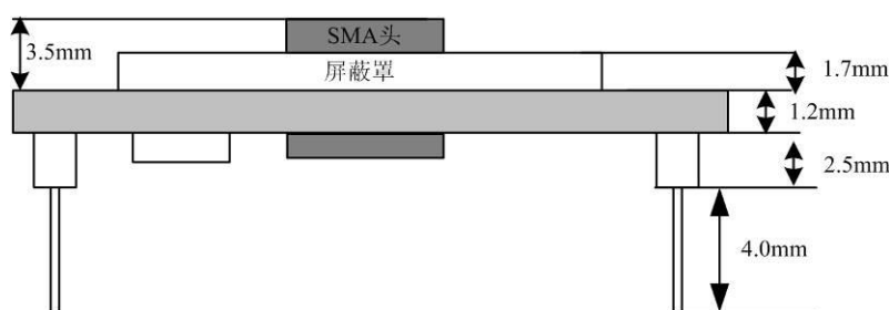
图 1-3 WLT2408Z 高度【侧视图】
